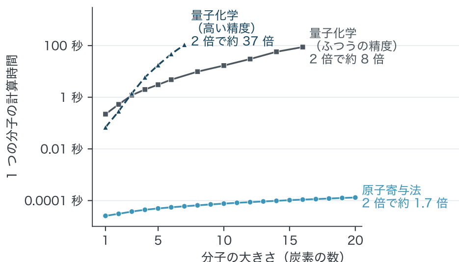
図 6-9 分子の大きさ（炭素の数）と、分子1個の計算にかかる時間。縦の目盛りは、1つ上がるごとに100倍になります。炭素1～2個の小さな分子では、計算の準備にかかる時間が目立つので、ふつうの精度の線が高い精度の線より上にあります。著者のノートパソコンのコア1つで測りました。
