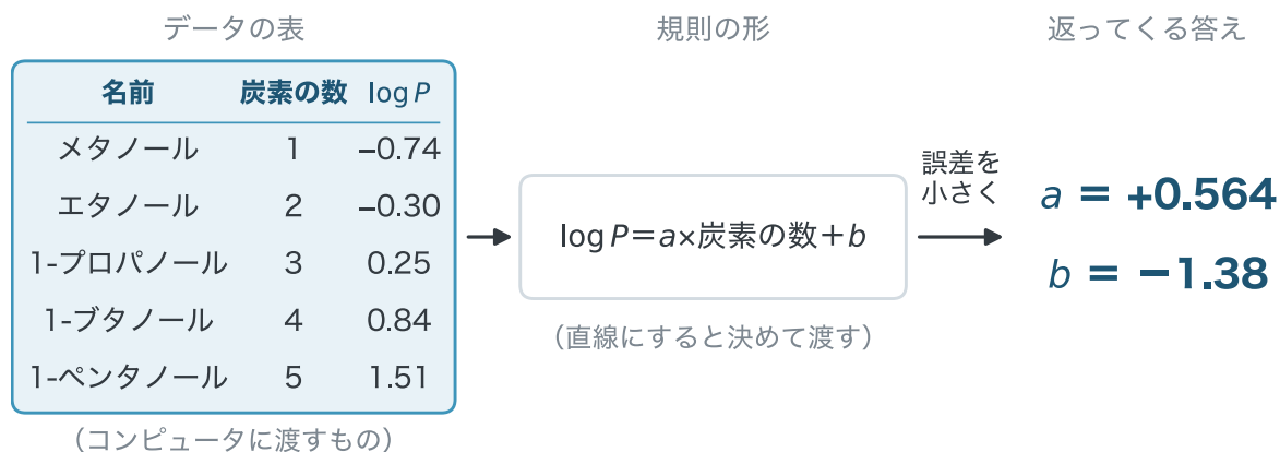
図 5-4 コンピュータに渡すもの (左と中) と、返ってくるもの (右)。
