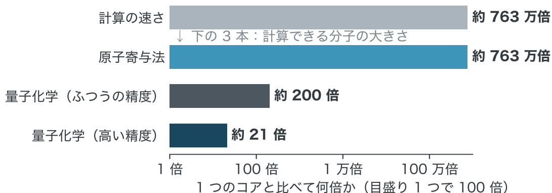
図 6-11 富岳のすべてのコアをむだなく使えたとき、コア 1 つと同じ時間で計算できる分子の大きさが何倍になるか。図 6-9 の増え方から見積もりました。
