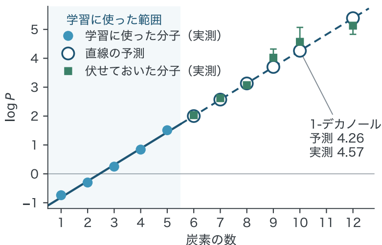
図 5-10 伏せておいた分子の予測と実測。学習に使った範囲の外では、直線を破線でのばしました。緑の四角の縦の線は、実測の不確かさの幅です (文献 5-2)。
