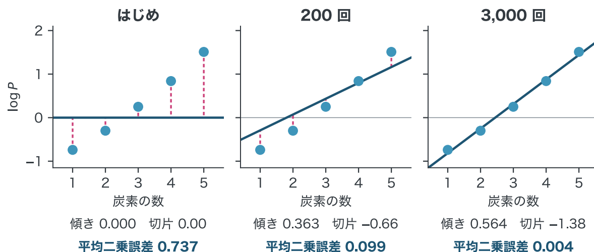
図 5-6 コンピュータの学習で、直線が丸に寄っていくようす。はじめ、200 回、3,000 回くり返したときの直線です。線と丸の意味は図 5-5 と同じです。
