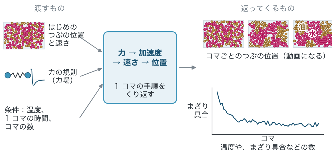
図 1-4 つぶを動かす計算で、コンピュータに渡すもの（左）と、返ってくるもの（右）。つぶの絵と線は、この章の水と油の計算（1.5 節）の出力です。
