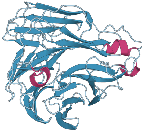
図 5-14 タンパク質の立体構造の例。第3章のノイラミニダーゼの鎖1本を、リボンのように描きました (PDB 2HU4 (文献 5-6))。ローズはらせん、青はシートと呼ばれる形です。
