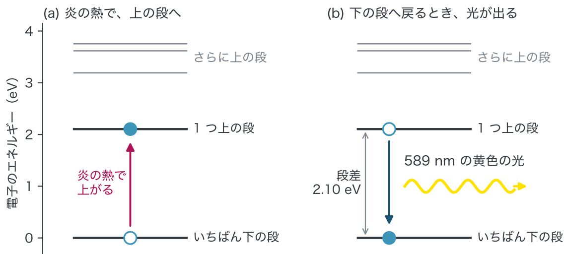
図 2-3 ナトリウム原子で、いちばん外側にある電子のエネルギー準位（横線）。丸が電子で、白抜きの丸は電子が移る前の位置です（文献 2-1）。
