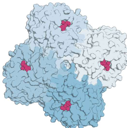
(b) ノイラミニダーゼの立体構造
