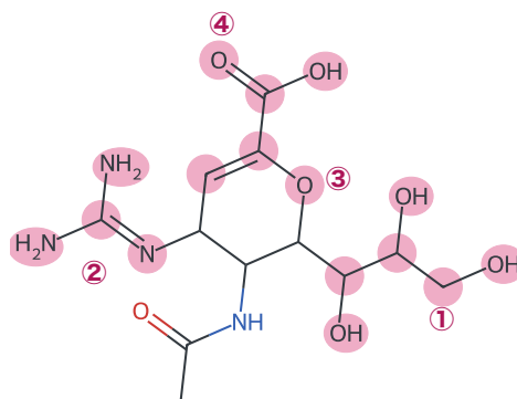
図 4-15 リレンザで書き換える 4 か所 (ローズ)。番号は左と同じです。
