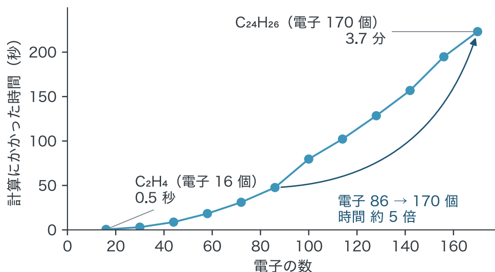
図 2-16 電子の数と、電子の雲を求める計算にかかった時間。炭素の鎖の分子（図 2-14 と同じ仲間）で、著者のパソコンの 1 コアで測りました。
