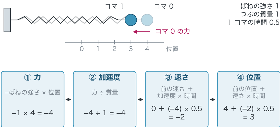
図1-5 手で1回、1コマ進める。上はつぶの位置(薄い丸がコマ0、濃い丸がコマ1)、下は4つの手順の計算です。
