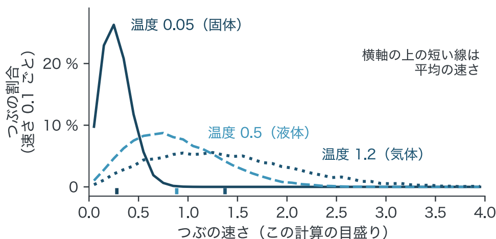
図 1-10 3つの温度での、つぶの速さの分布（図 1-9 と同じ計算の出力）。
