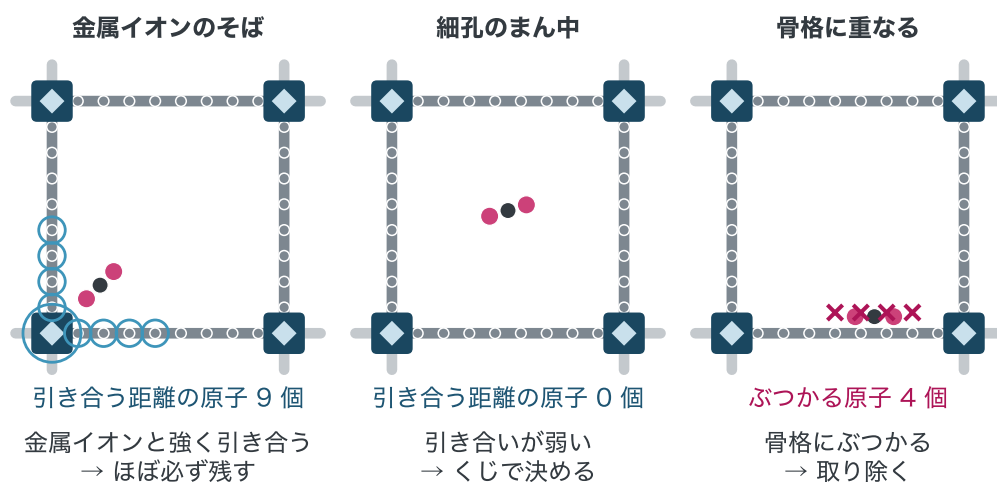
図 終-5 細孔の 3 か所に CO 2 を置いてみる（考え方を見せるための、平面の細孔の模型）。青い輪は、置いた CO 2 と引き合う距離にある骨格の原子、× は CO 2 とぶつかる原子です。
