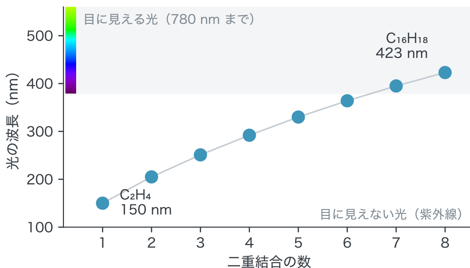
図 2-14 二重結合と単結合が交互に並んだ炭素の鎖の、段差に見合う光の波長 (本書で計算した値)。左の色の帯は目に見える光の範囲で、帯の色は、その波長の光の色です (分子そのものが見える色ではありません)。
