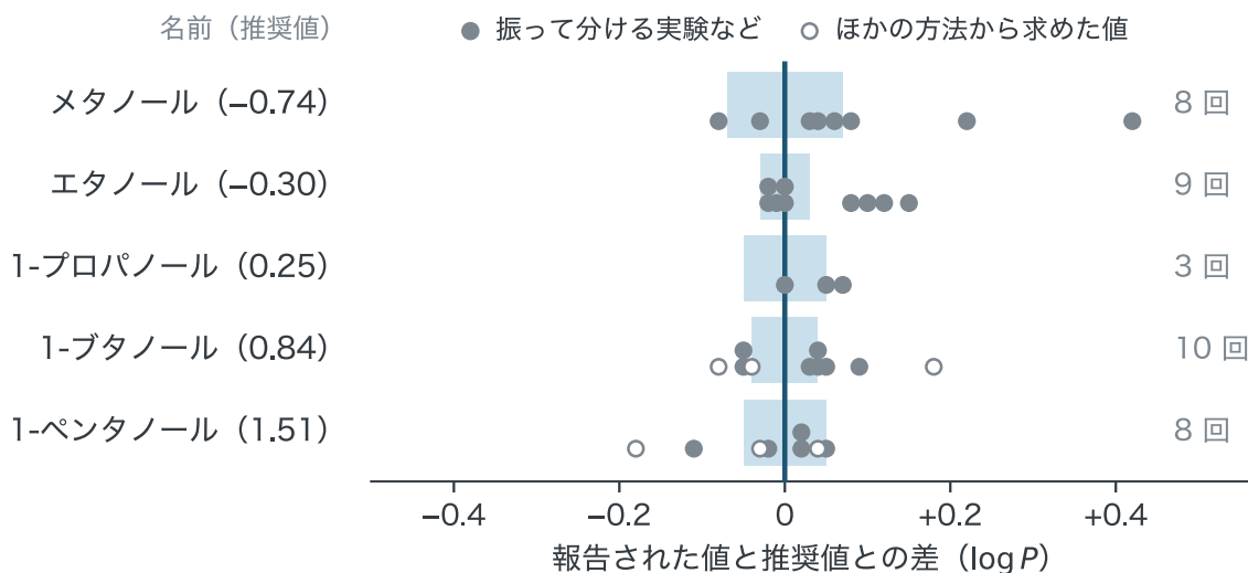
図 5-1 直鎖のアルコール 5 つについて報告された \log P の値。横の位置は、それぞれの値と推奨値との差です。同じ値の丸は縦に積みました。青い縦線が推奨値、淡い青の帯が不確かさの幅です。原典で疑わしいとされた値は除きました (文献 5-2)。
