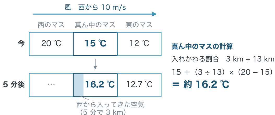
図 序-3 手で 1 回、マスの気温を 5 分進める。淡い青の部分が、5 分のあいだに西のマスから入ってきた空気です。風が気温を運ぶことだけを考えた、簡単にしたモデルです。
