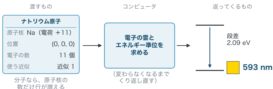
図 2-6 量子化学計算で、コンピュータに渡すもの（左）と、返ってくるもの（右）。右の段差と波長は、本書で計算したナトリウム原子の値です。近似 1 は図 2-17 と同じです。
