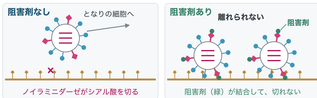
図 3-3 ノイラミニダーゼのはたらき（左）と、阻害剤のはたらき（右）。× は、ノイラミニダーゼが切ったシアル酸です。
