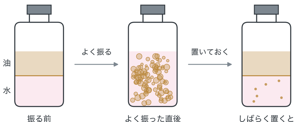
図 1-1 水と油を入れたびんを振る実験。びんと滴は、形を簡単にした絵です。
