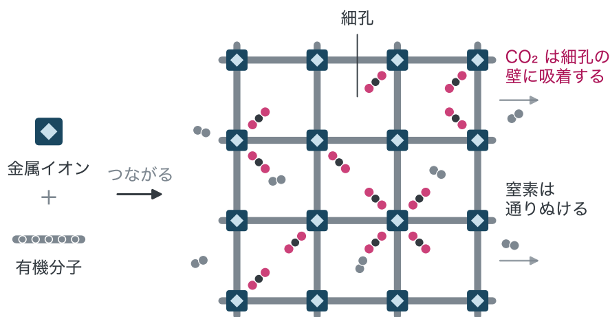
図 終-2 MOF のつくりと、細孔に CO 2 がとどまるようす（模式図）。紺の四角が金属イオン、灰色の棒が有機分子です。CO 2 は 3 つの丸（O・C・O）、窒素は灰色の 2 つの丸で描いています。
