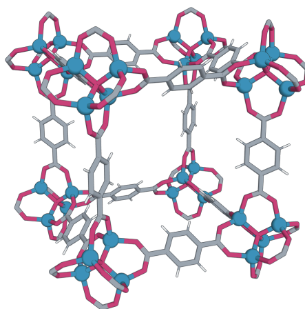
(b) MOF-5 の結晶構造
