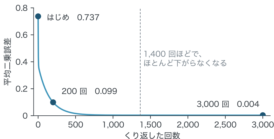
図 5-7 くり返した回数と、平均二乗誤差。
