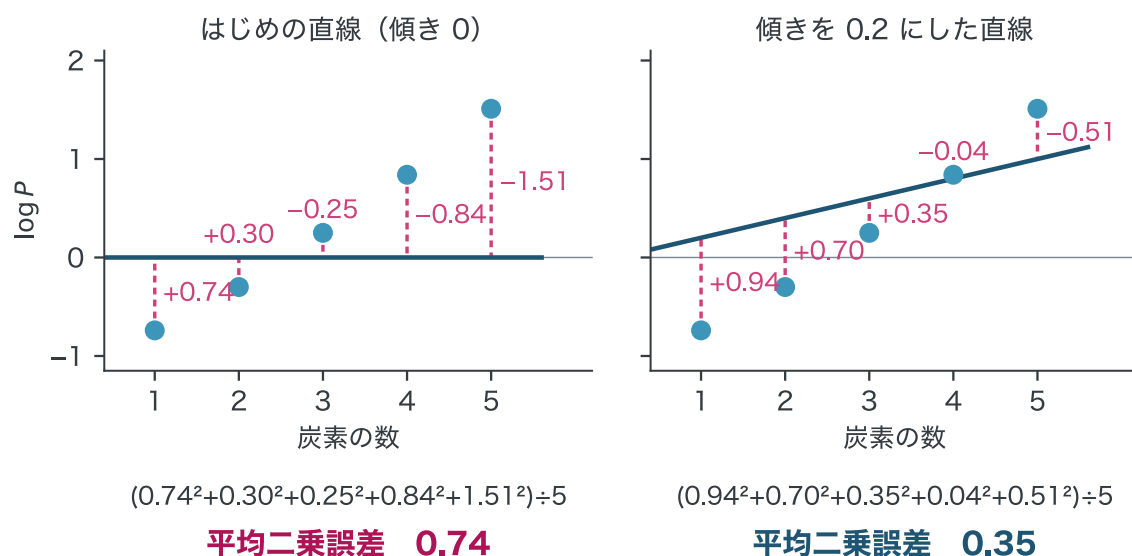
図 5-5 手で 1 回、直線を動かす。丸が実測、紺の線が直線、ローズの点線と数が予測の誤差（予測 - 実測）です。下は平均二乗誤差の計算です。
