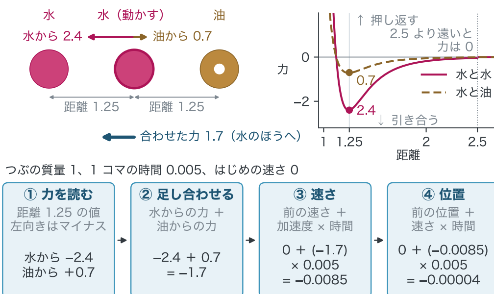
図 1-13 手で 1 回、水をつぶを 1 コマ進める。左上は 3 つのつぶと、真ん中の水をつぶにはたらく力（矢印の長さが力の大きさ）、右上はつぶどうしの力と距離の関係（図 1-3 の右と同じ式）、下は 4 つの手順の計算です。
