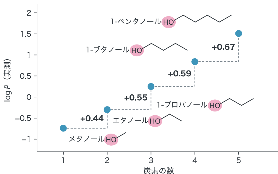
図 5-2 直鎖のアルコールの、炭素の数と \log P (実測) の散布図。名前の横は骨格構造式で、O-H の O をローズで塗りました。点線の階段の数は、炭素が 1 個増えたときの \log P の増加分です (文献 5-2)。
