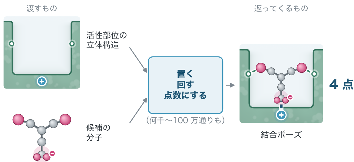
図 3-10 ドッキングで、コンピュータに渡すもの (左) と、返ってくるもの (右)。活性部位と分子は、考え方を見せるための簡単な絵で、線と玉の意味は図 3-6 と同じです。
