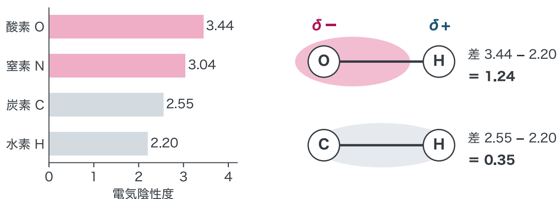
図 2-11 H・C・N・O の電気陰性度 (左) と、O-H・C-H の結合の電荷のかたより (右)。右の楕円は結合の電子を表し、O-H では O の側に寄っています (文献 2-3)。
