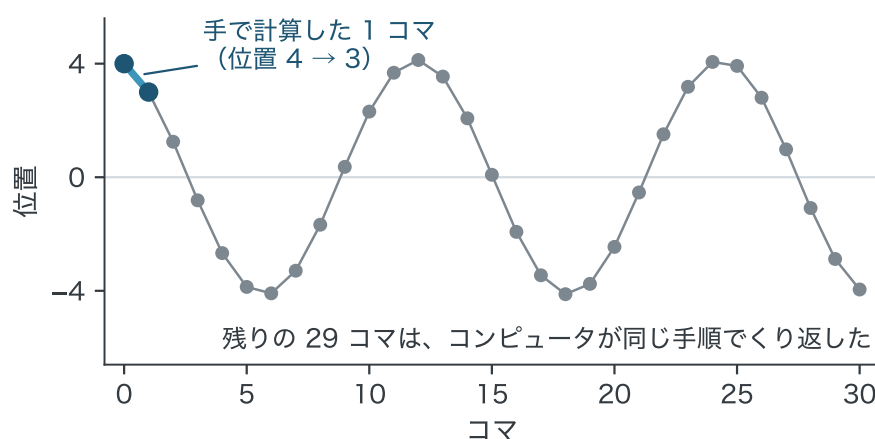
図 1-6 図 1-5 の手順を 30 回くり返したときの、つぶの位置。
