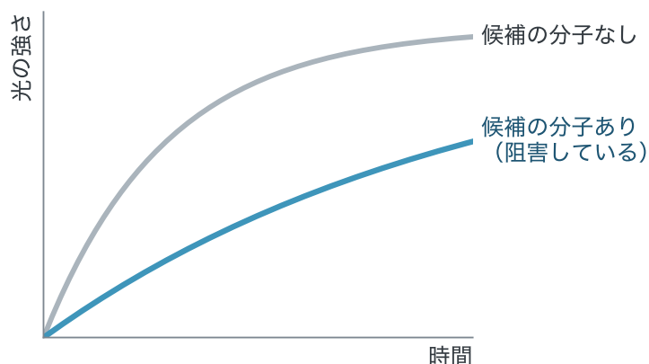
図 3-4 阻害の実験で、時間がたつにつれて光が強くなるようす。考え方の図なので、目盛りの値は描いていません。
