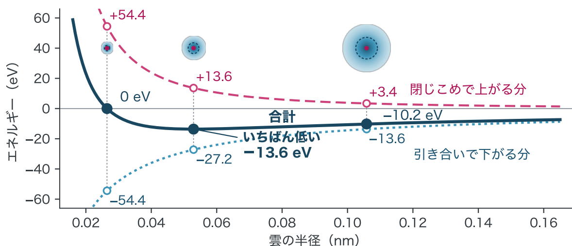
図2-7 水素原子の電子の雲の半径と、エネルギー（本書で計算した値）。丸が、手で試した3通りの大きさで、丸の横の数がそれぞれの値（eV）です。丸の上の絵は、その大きさの雲の切り口で、点線の円が雲の半径です。
