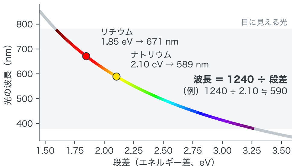
図 2-4 段差と光の波長の関係。曲線の色は、その波長の光の色です。灰色の部分は、目に見えない光です。丸は、ナトリウムとリチウムの実測の値です（文献 2-1）。
