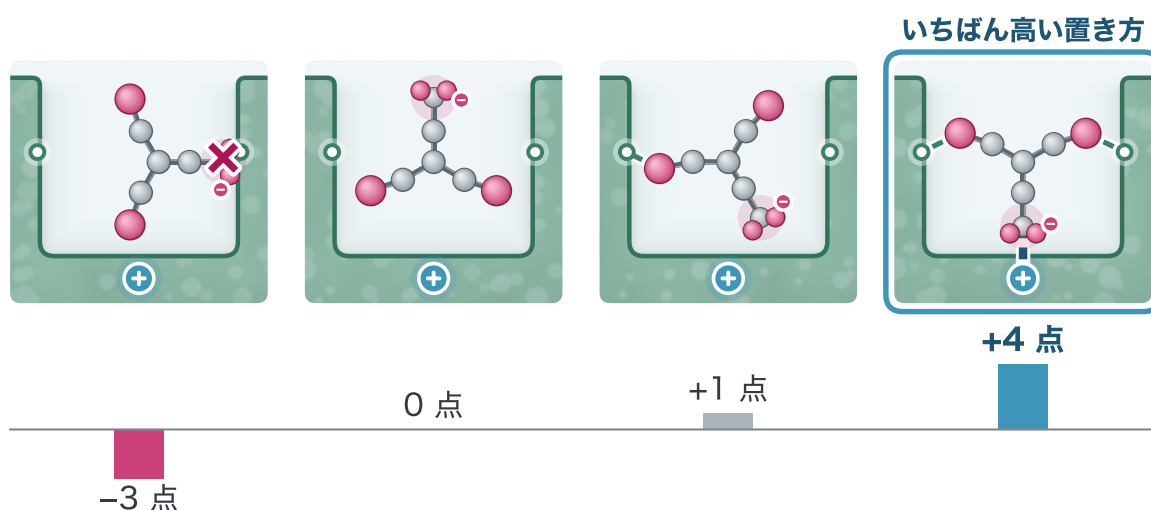
図 3-12 同じ分子の、置き方のちがう 4 通りと、その点数 (点数の低い順)。× は壁にぶつかった原子です。
