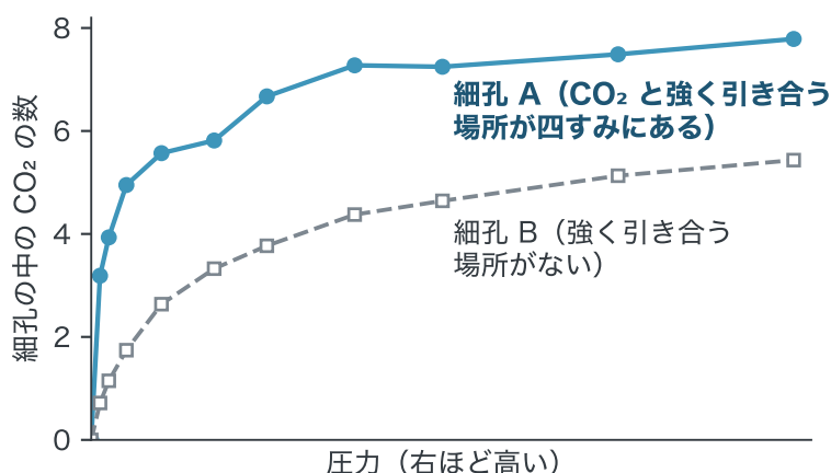
図 終-6 この本の模型で計算した、2つの細孔の吸着等温線。縦軸は、細孔に入っている \text{CO}_2 の数の平均です。考え方を見せるための模型で、本物の MOF の値ではありません。横軸の目盛りの値は描いていません。
