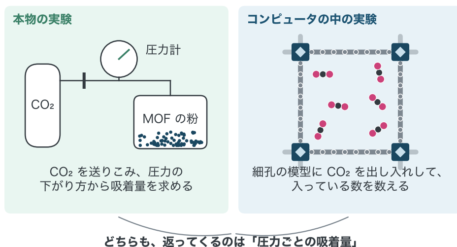
図 終-4 同じ問いに答える、本物の実験（左）とコンピュータの中の実験（右）。左は装置を簡単にした絵です。右の \text{CO}_2 の並びは、この本の模型で計算したものです。
