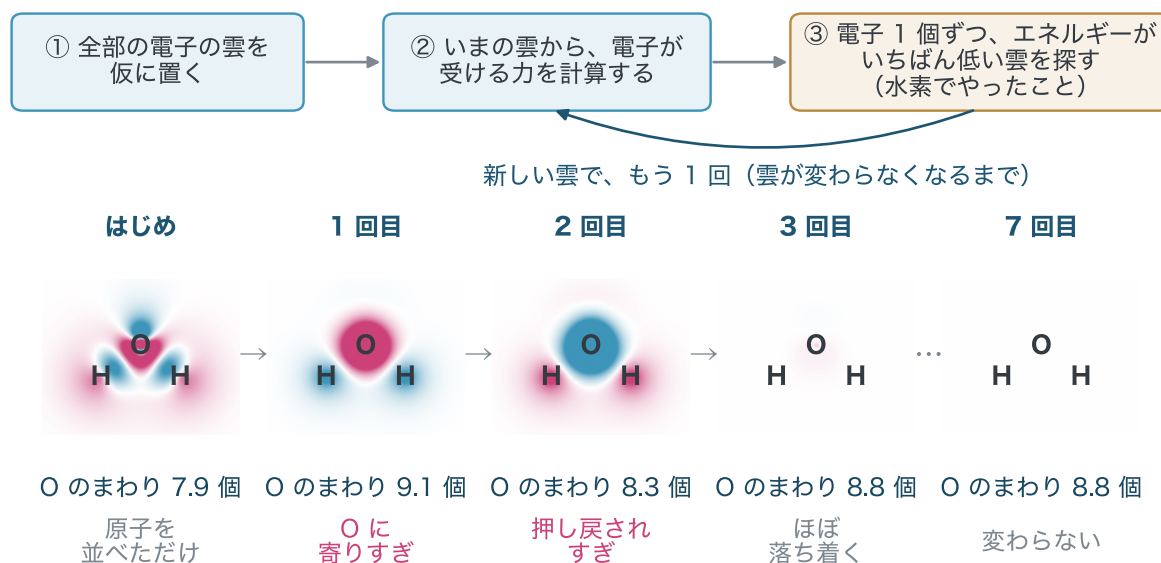
図 2-9 電子の雲を求めるくり返し (上) と、水分子で計算したときの回ごとの雲 (下。本書で計算した値)。下の段は、各回の雲と最後の雲との差を、分子の平面での切り口で塗りました。ローズは最後の雲より電子が多い所、青は少ない所です。Oのまわりの電子の数は、電子10個を原子ごとに分けた数で、分け方によって少し変わります。
