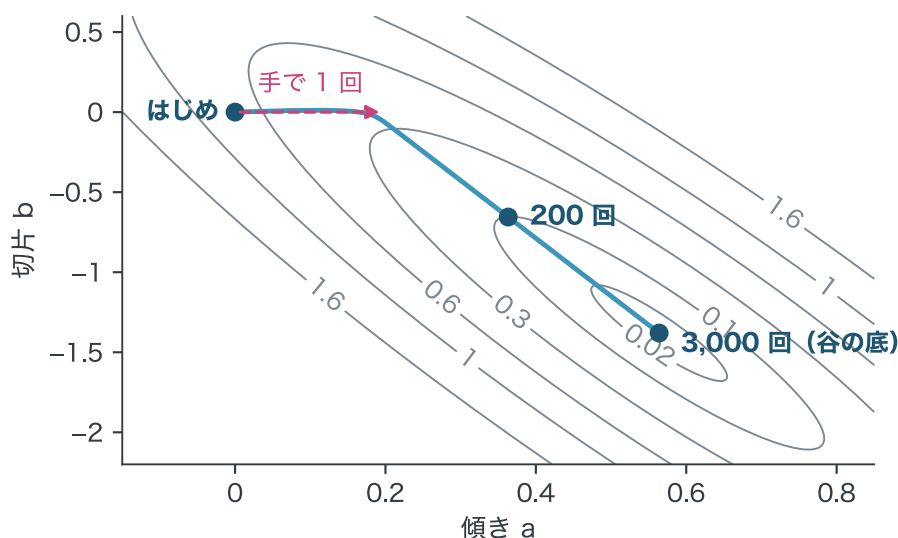
図 5-8 誤差の地図と、学習がたどった道。横が傾き a 、縦が切片 b で、灰色の線は平均二乗誤差の等高線（数は平均二乗誤差）です。青の線が、コンピュータの学習でたどった道、ローズの矢印が、手で1回動かした分です。
