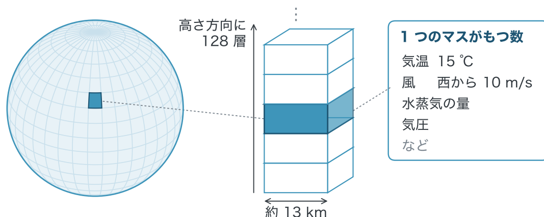
図 序-2 大気を格子のマスに区切ったようす（模式図）。地球の上の格子の線は、本物（約 13 km 間隔）よりずっと粗く描いています。マスの中の値は例です（文献 序-2）。
